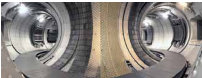
Installation Tore Supra à Cadarache
